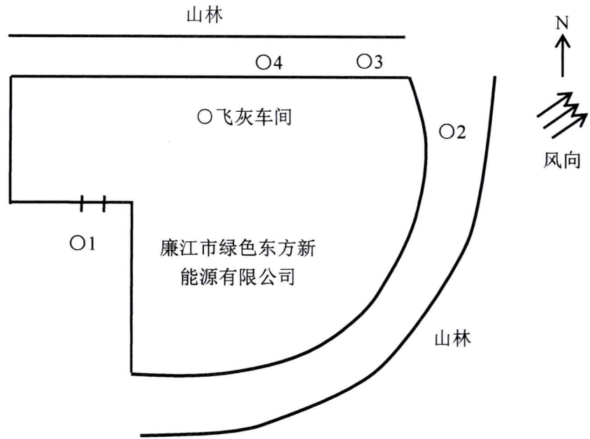
图1 检测点位示意图 (○表示无组织废气检测点)
